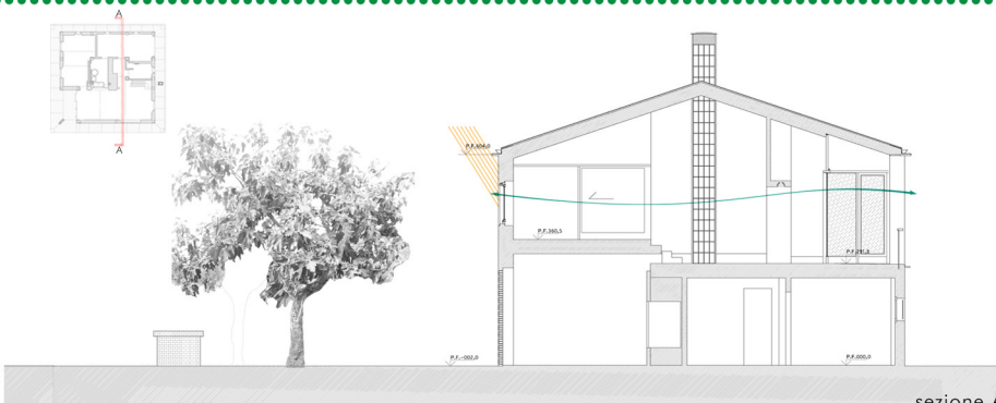
sezione AA'
