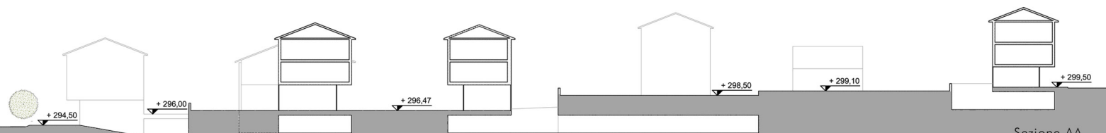
Sezione AA
